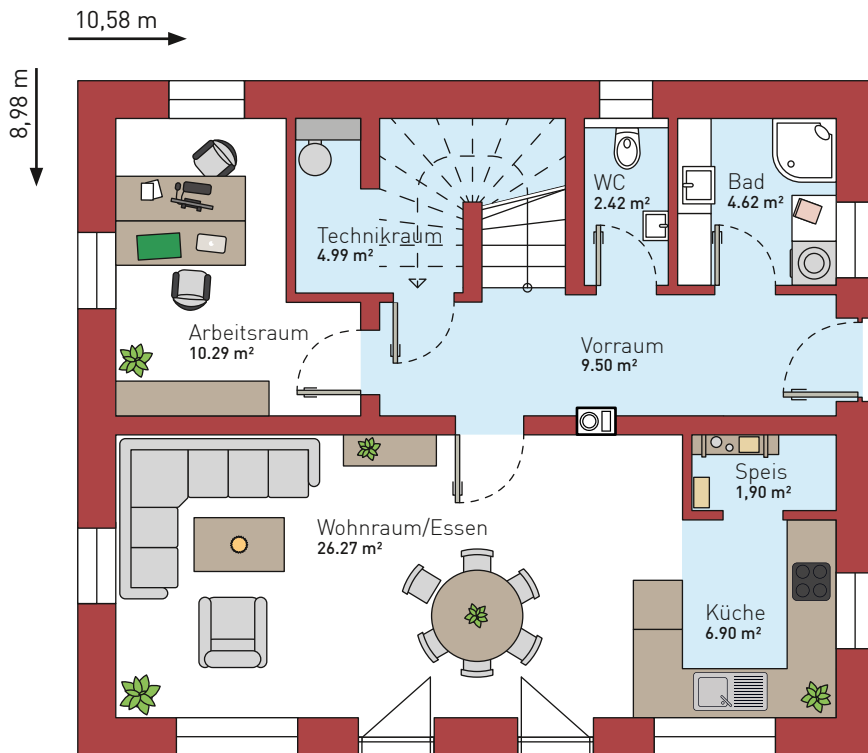
Erdgeschoß Maßstab 1:100
