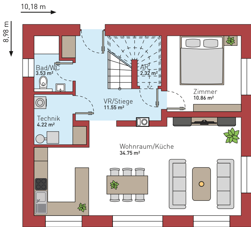
Erdgeschoß Maßstab 1:100
