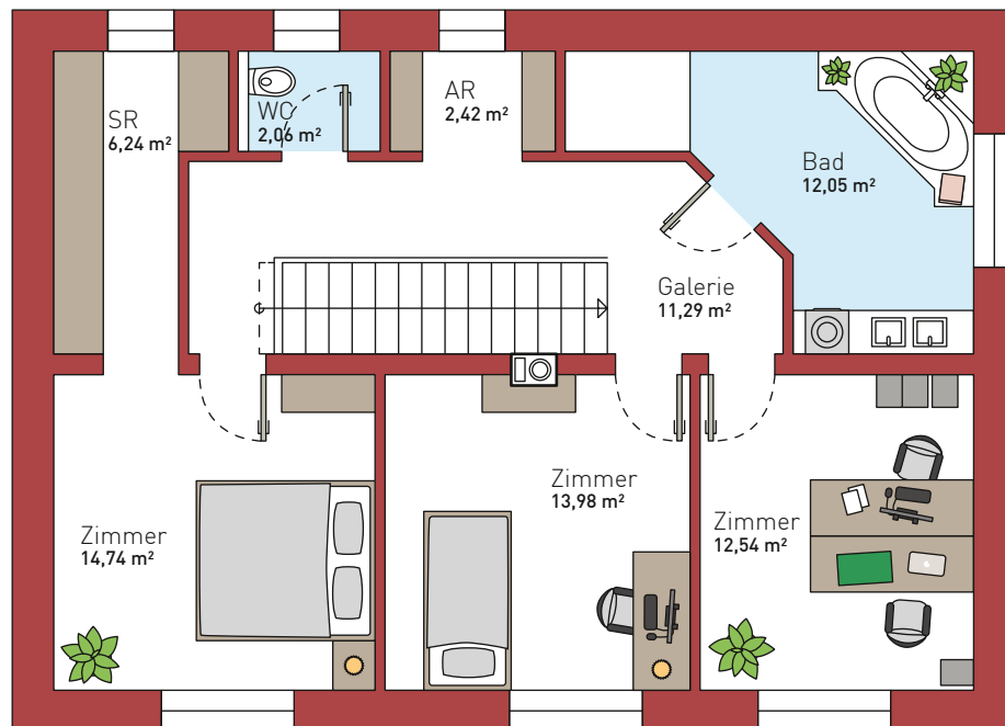
Obergeschoß
