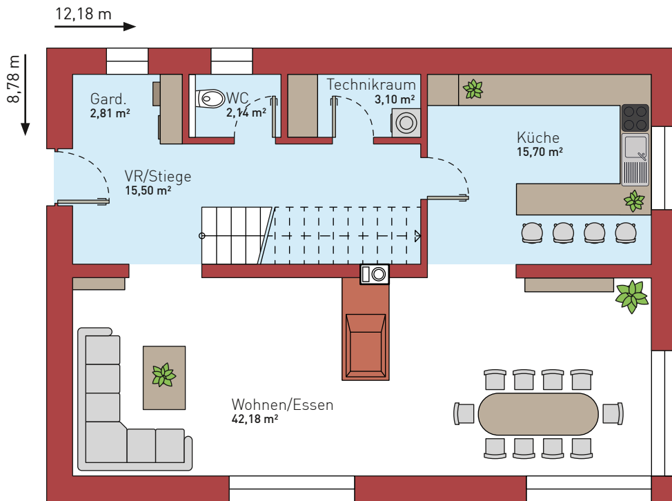
Erdgeschoß Maßstab 1:100
