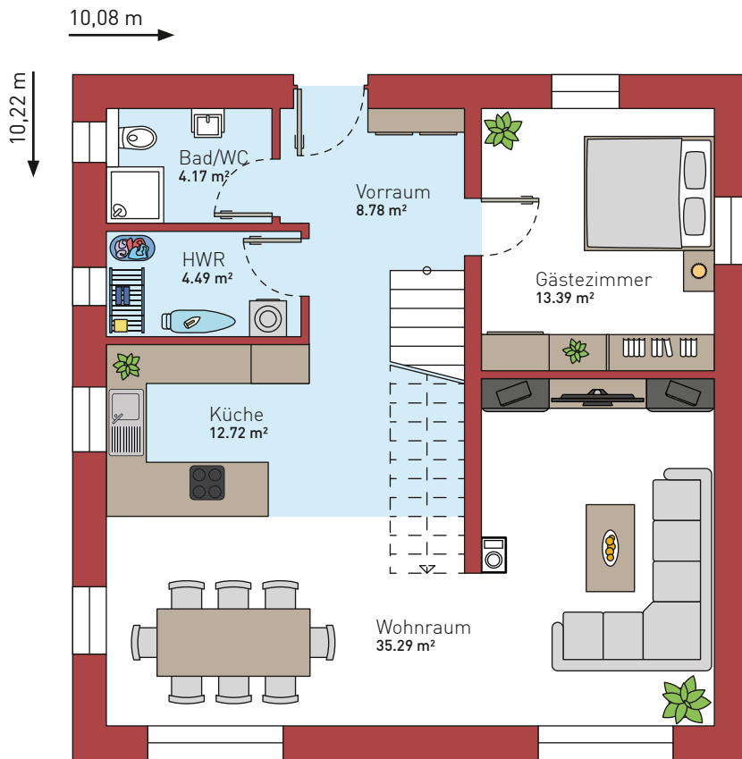
Erdgeschoß Maßstab 1:100
