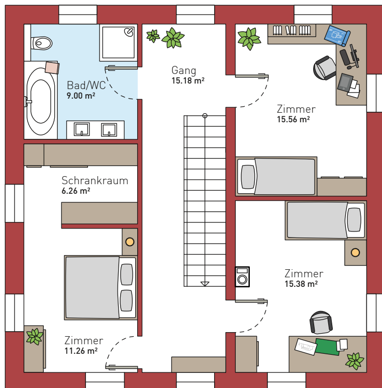
Obergeschoß
