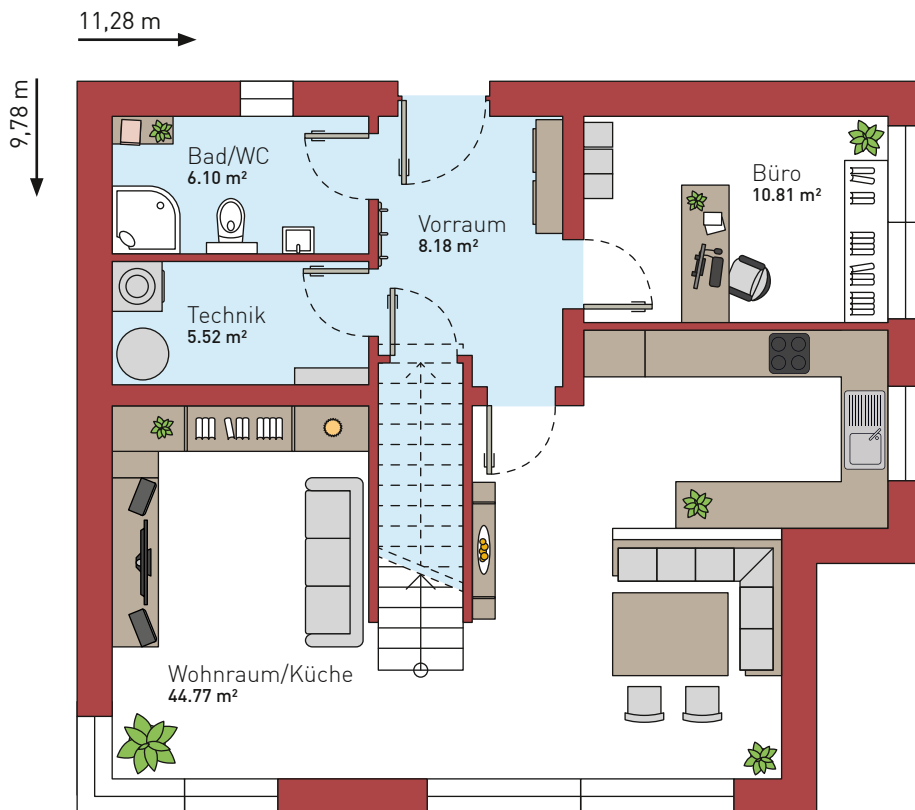
Erdgeschoß Maßstab 1:100
