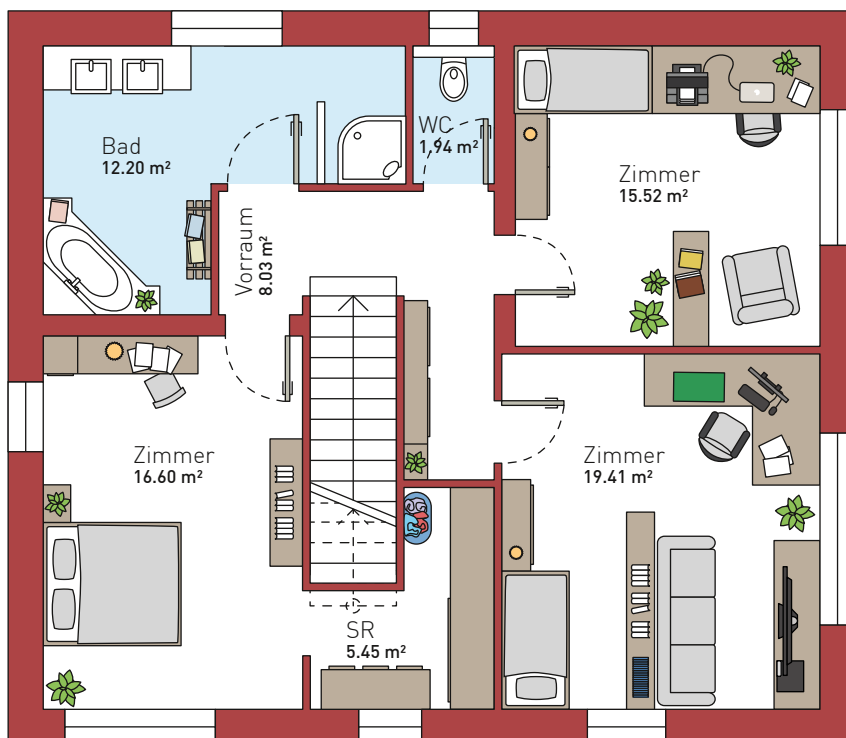
Obergeschoß
