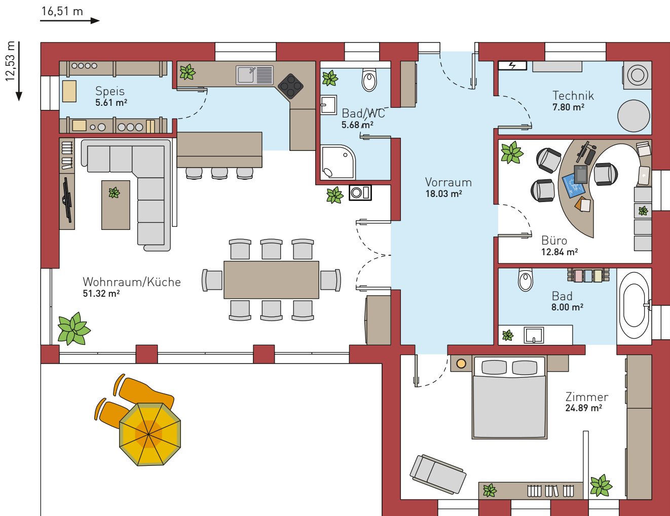
Erdgeschoß Maßstab 1:100
